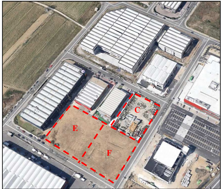
Foto aeree con individuazione zona localizzazione lotti P.I.P.
